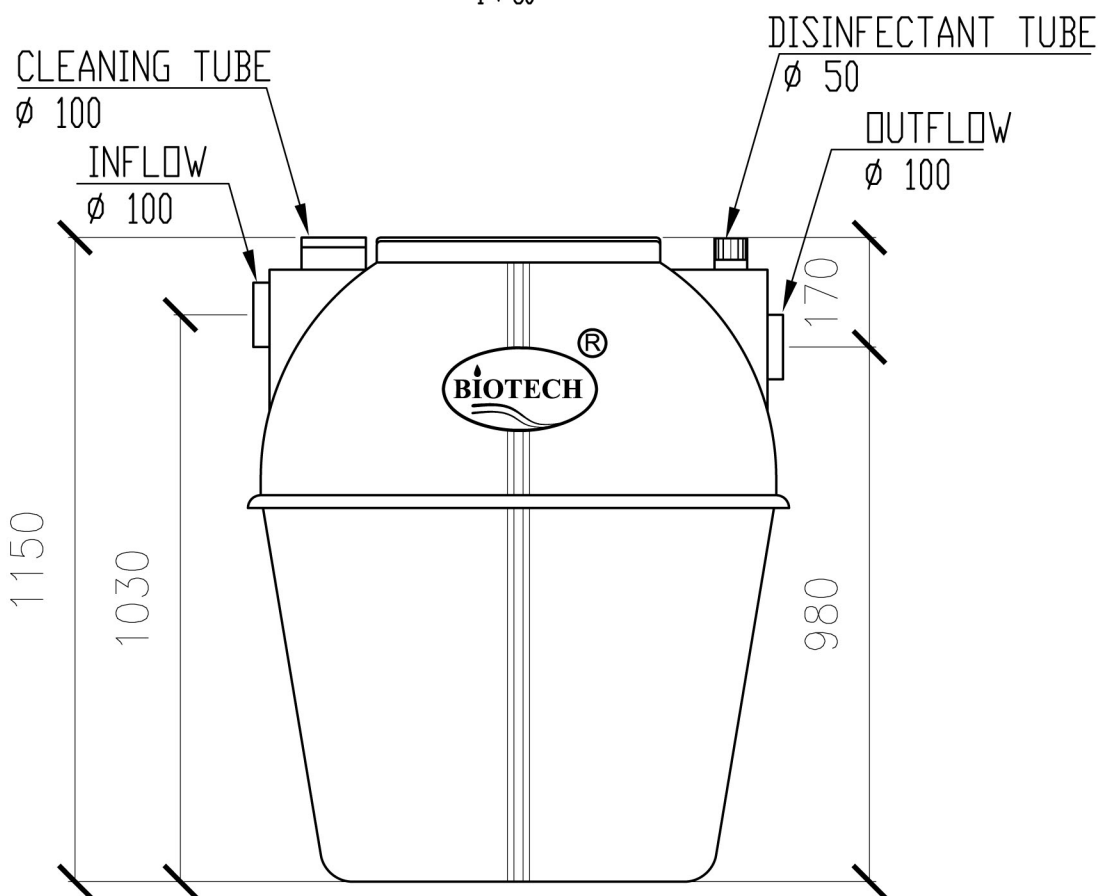
TAMPAK SAMPING 1 : 30
