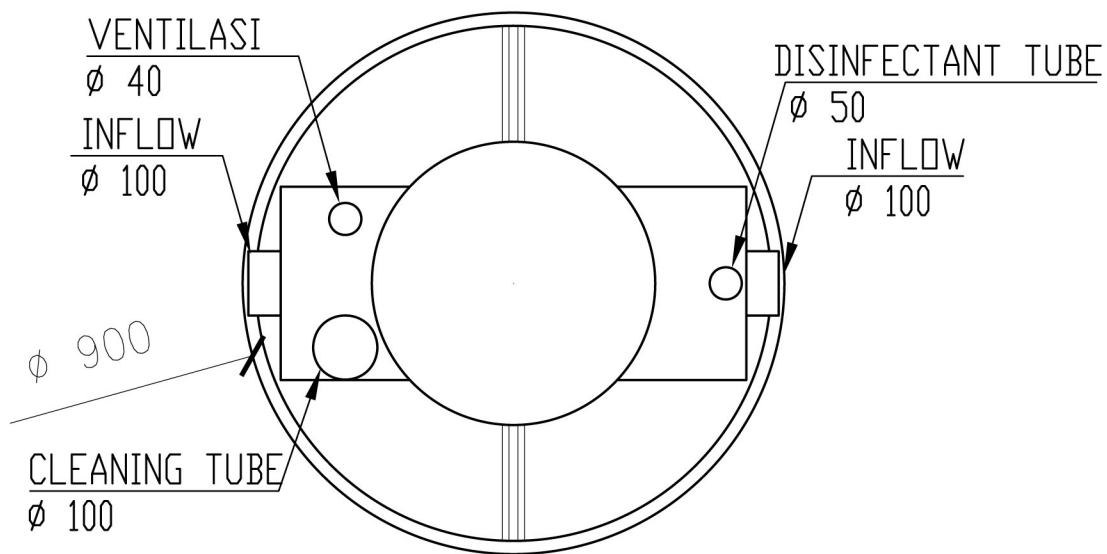
TAMPAK ATAS 1 : 30
